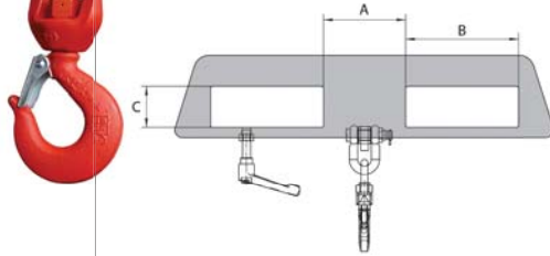
Dimension intérieure des fourreaux (mm) (Croquis type PAF02) Fork sleeve inside dimensions (drawing Type PAF02)
